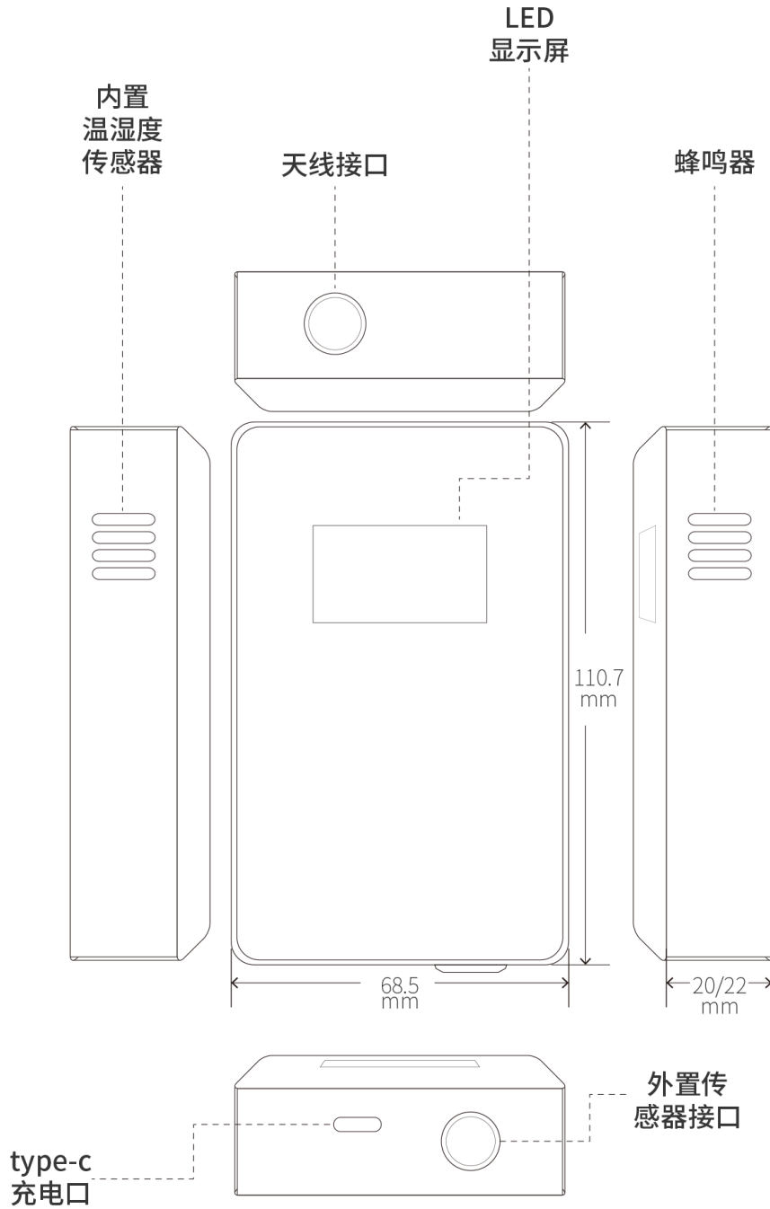
尺寸图
